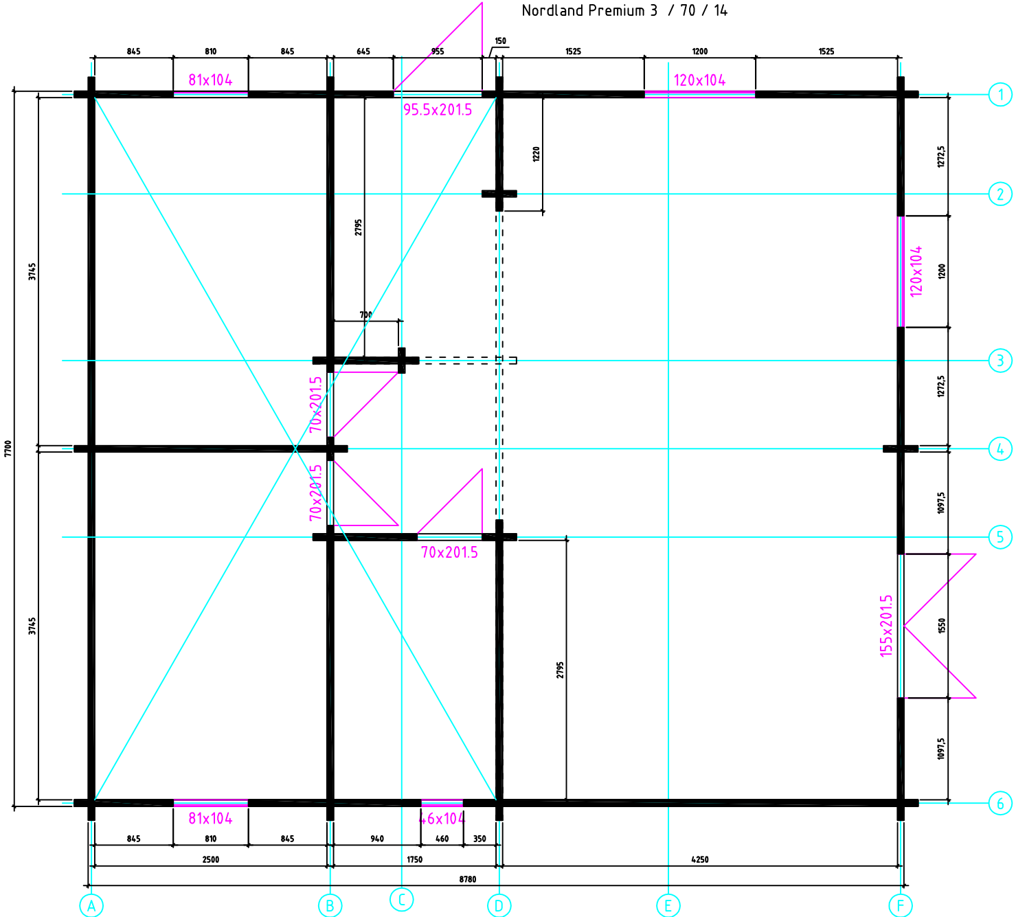
Grundplan
