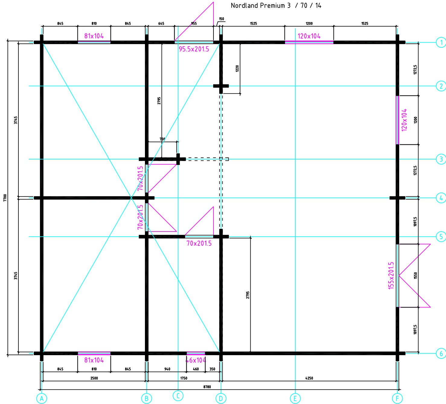
Grundplan
