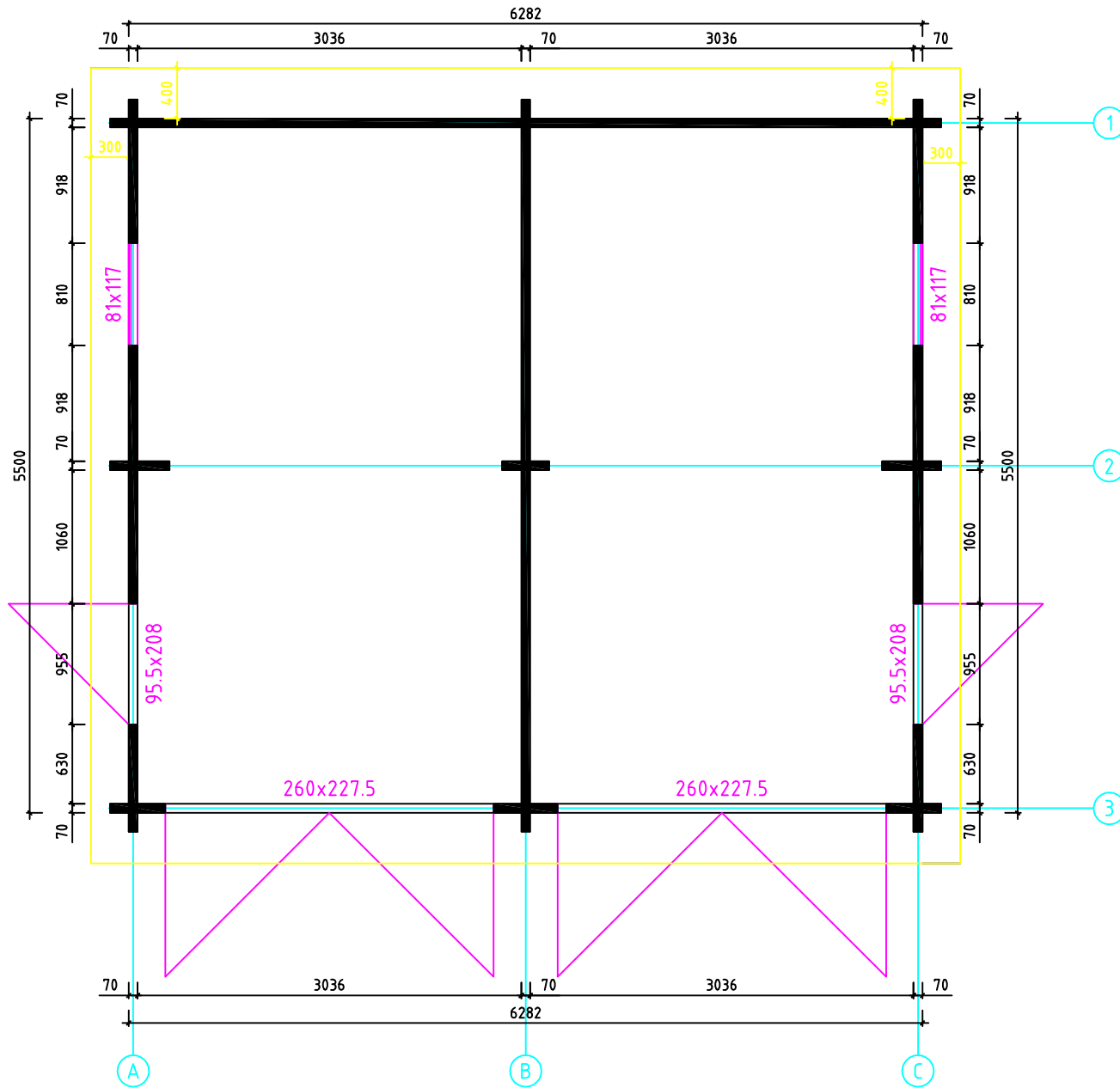
Grundplan Doppelgarage
