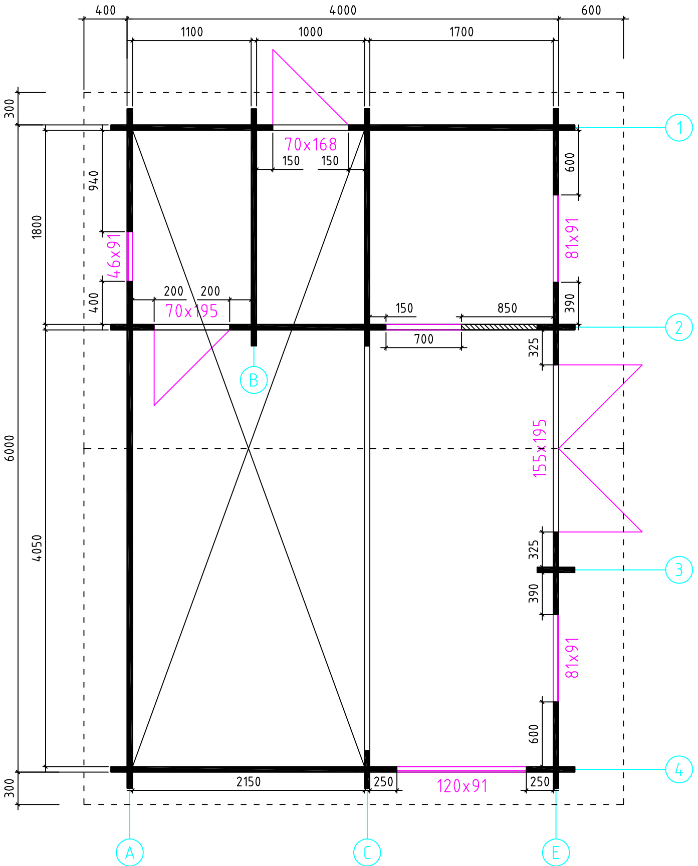
Grundplan
